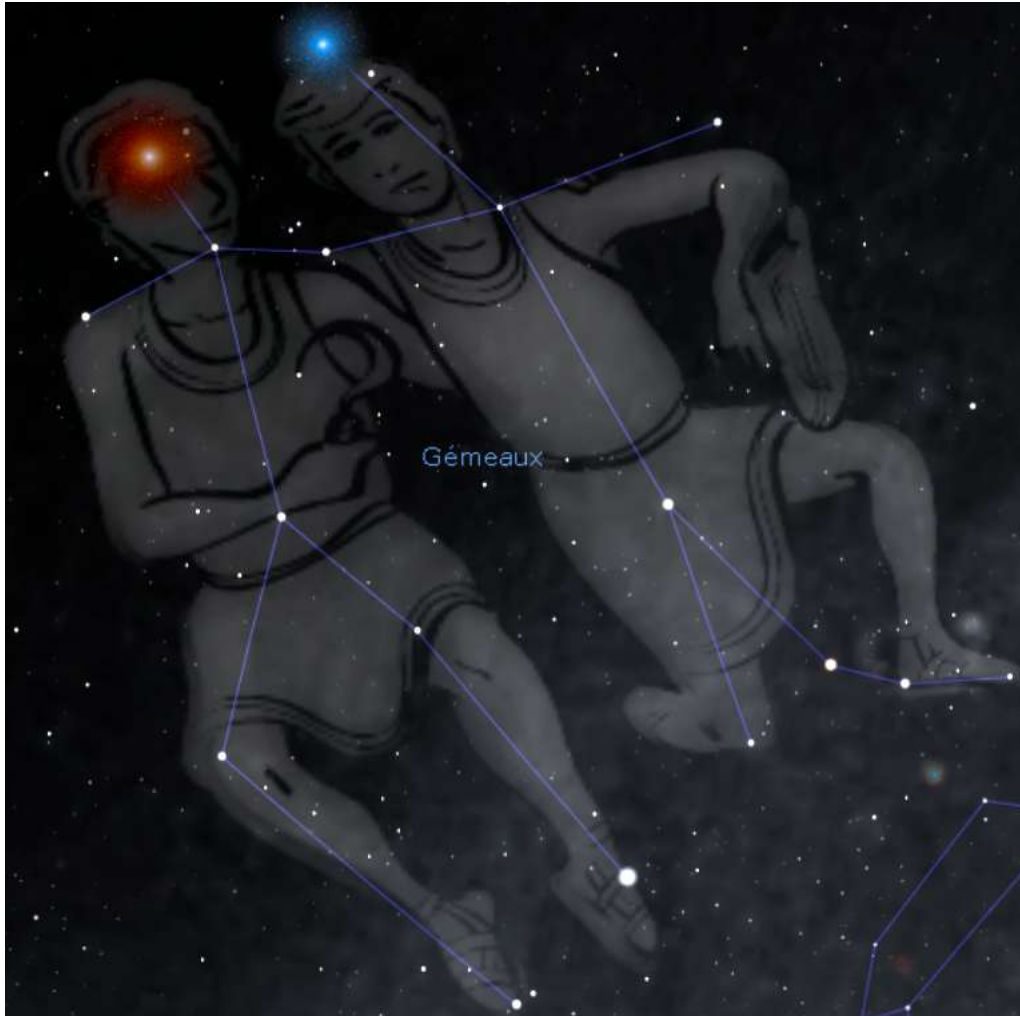
De gauche à droite : Pollux et Castor - Stellarium
